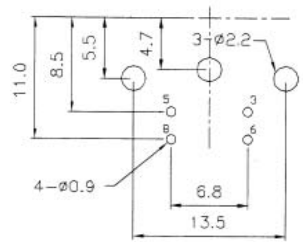
P.C.B LAYOUT(±0.1) (BOTTOM VIEW)
